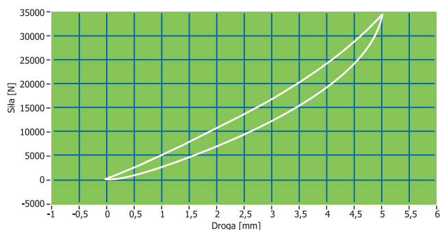
AMORTYZATOR PŁASKI MDL 90L
