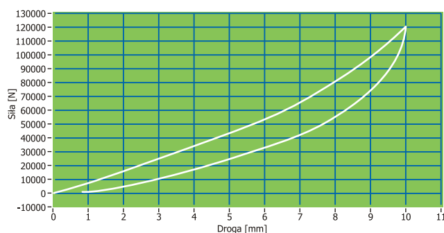
AMORTYZATOR PŁASKI MDL 180L
